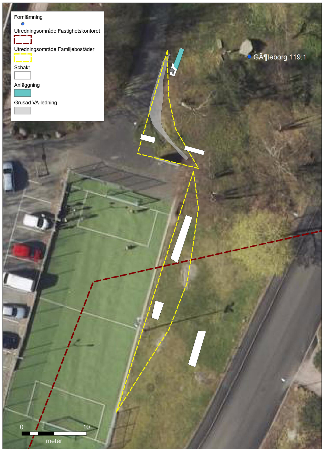
Schakt och anläggningar inom kompletterande yta vid hållkistan Göteborg 119. Skala 1:300.
